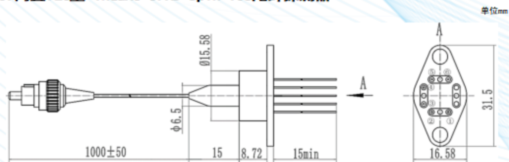
底视图
