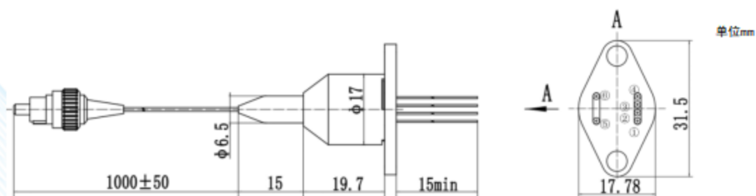
底视图
